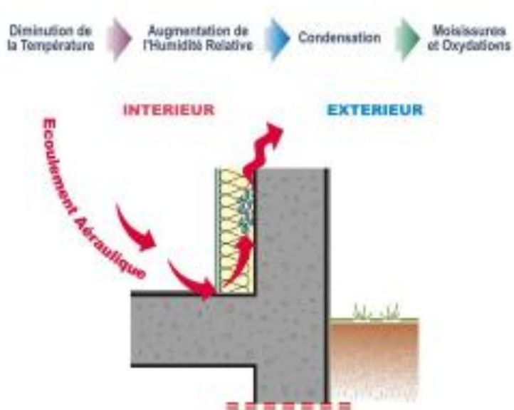
Figure 5 : Illustration de la condensation dans les parois.
